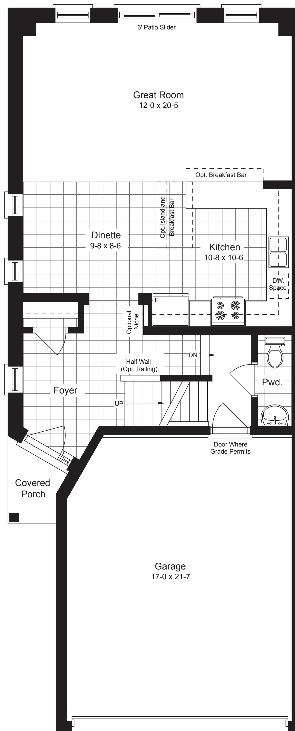
MAIN FLOOR - M1
